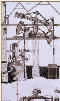
(9) Ohňový (parný) stroj na čerpanie vody z bani, polovica 18. storočia. Prvý takýto stroj postavili v Novej Bani v roku 1722
